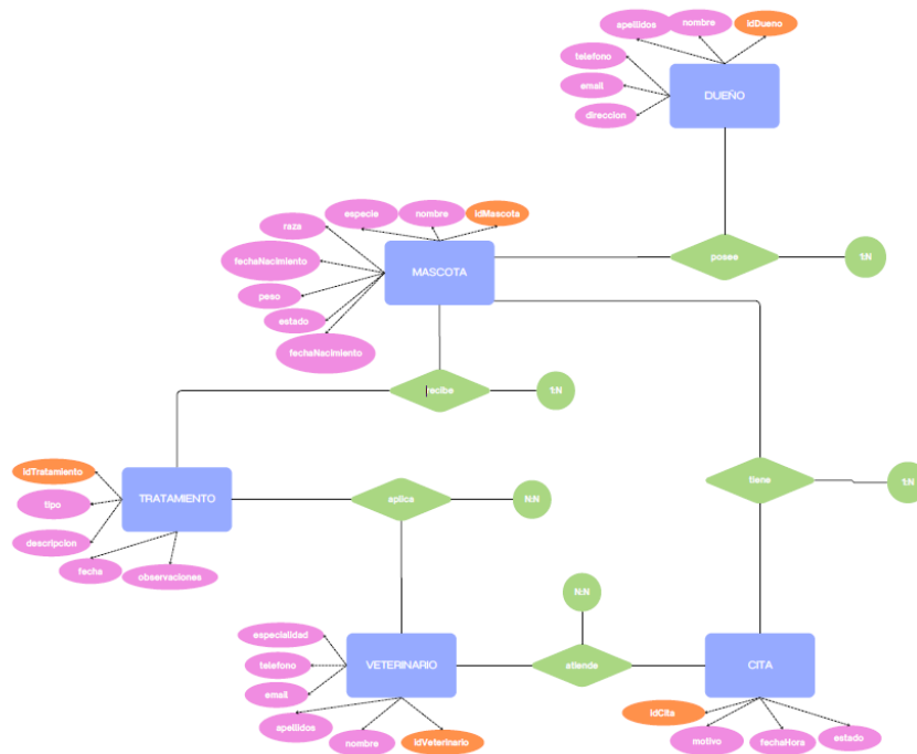
Diagrama de entidad-relación: VeteriApp
